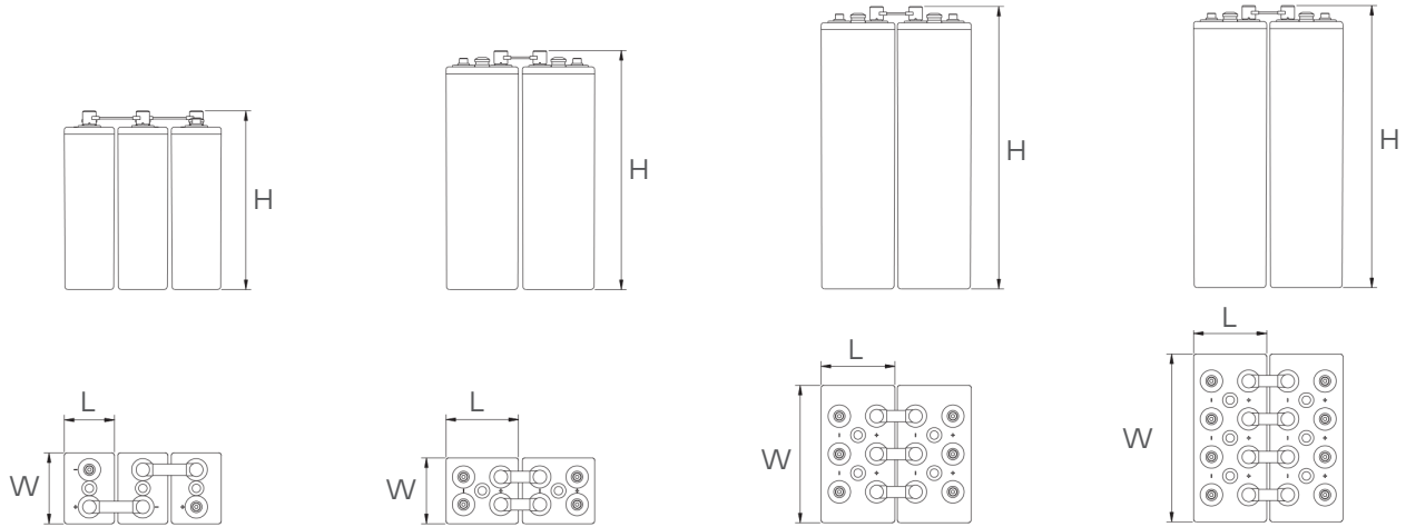
NSB 6 OPzV 300 - NSB 6 OPzV 600
