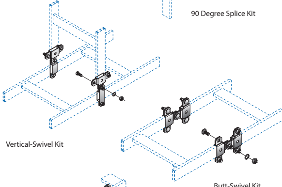
Butt-Swivel Kit
